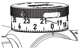
Compteur de rotations du CDS-ZL 2 (2ème rotation)
