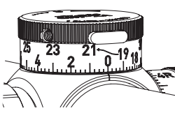
Cadran d'élévation du CDS-ZL 2 (en position verrouillée)
