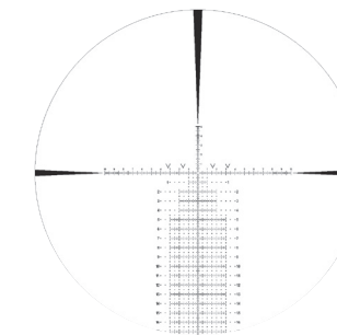
CCH Reticle
